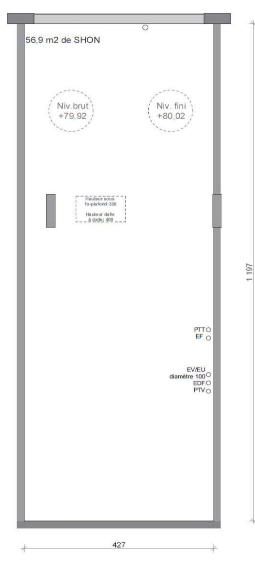
Plan brut du local
